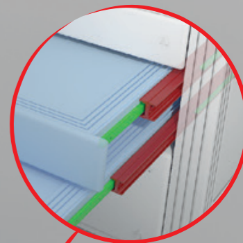
> Ouverture de tiroir Drawer extraction
