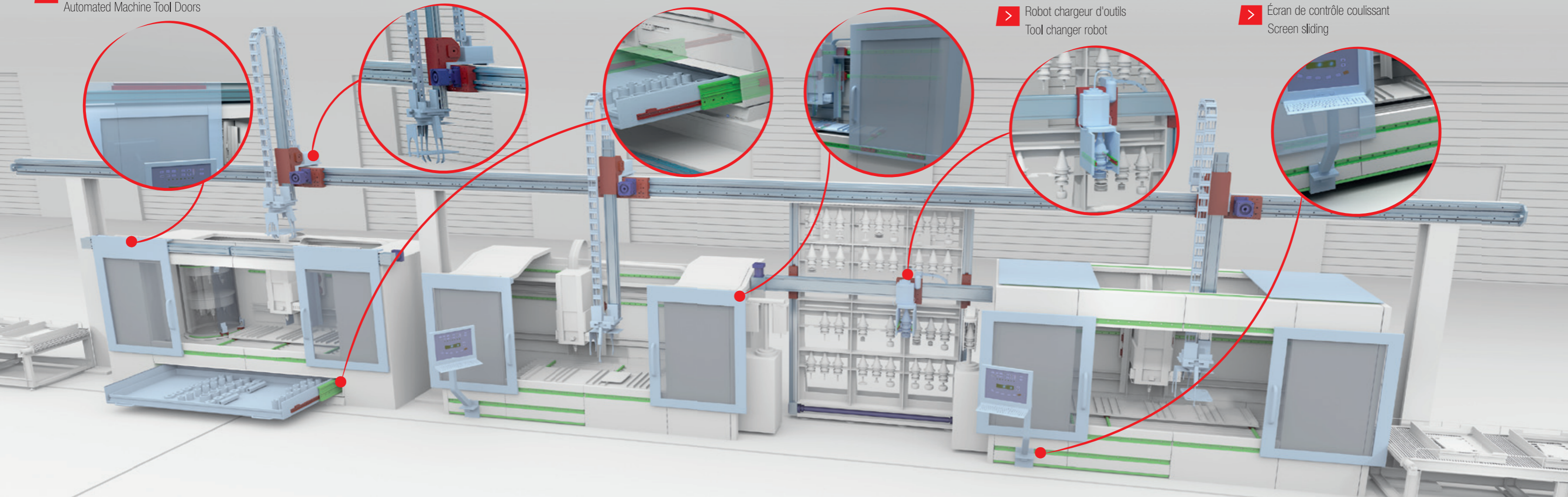
> Chargement et déchargement de pièces usinées Loading & unloading of the machined piece
